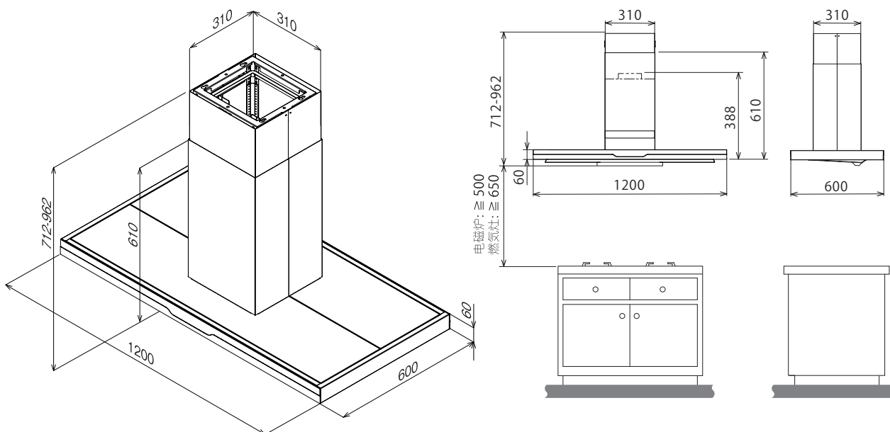
尺寸图 [mm]
